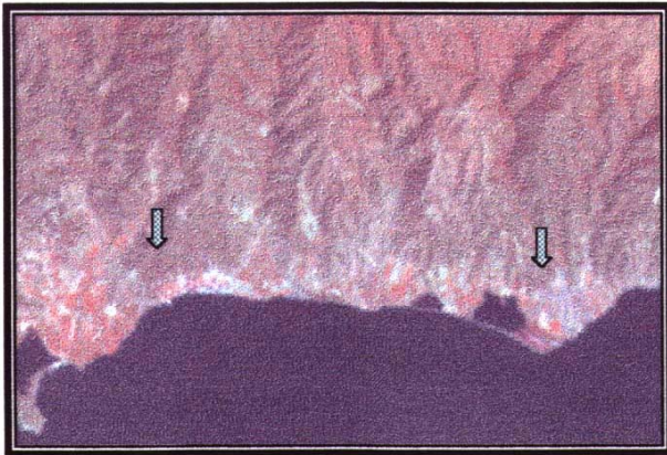
Εικ.2. Τμήμα της Δορυφορικής Εικόνας LANDSAT 5, TM, Ψευδέγχρωμης, 4-7-2 (RGB), Νότιας Αργολίδας. Κατά μήκος της νότιας ακτής των Αδέρων παρατηρείται Ρήγμα παράλληλο με την ακτή. Κατά μήκος αυτού παρουσιάζονται κώνοι κορημάτων, λιμνοθάλασσες και αλλούβια ή απότομες ακτιές. Τα βέλη δείχνουν τη θέση που διέρχεται το ρήγμα. Part of the LANDSAT 5, TM, satellite image, false color composite, 4-7-2 (RGB), of Northern Argolis Peninsula. Along the northern coastline of Adheres Mountain, a fault parallel to the coastline is observed. Along the fault, scree, lagoons, alluvials and steep coastline can be viewed. The arrows indicate the fault line.
